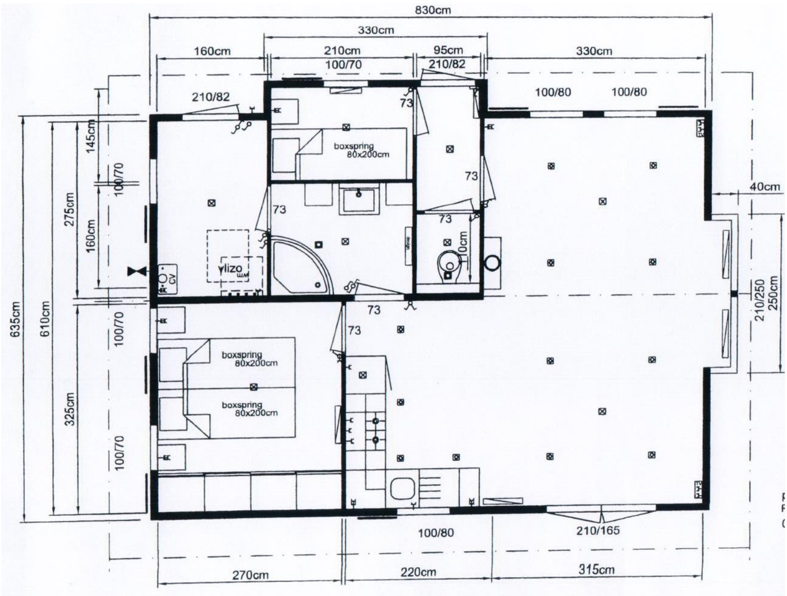
Plattegrond Parkwoning
